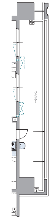
2階・3階バルコニー部分図 scale ≒ 1/150
